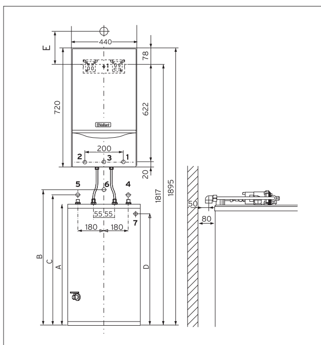
VU INT 126/3-5, 186/3-5, 246/3-5, 376/3-5, 256/3-3 + zásobníkový ohřívač uniSTOR VIH R
