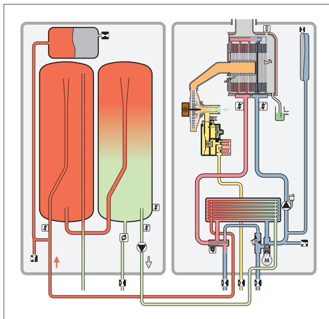
Dobíjanie zásobníka v zostave VUI bez odboru teplej vody
