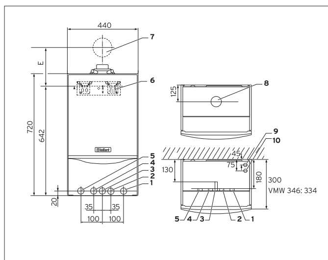
VUW INT 236/3-5, VUW INT 226/3-3
