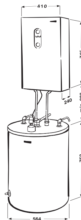
Rozmerový náčrtok zostavy Raja + B 120 S
