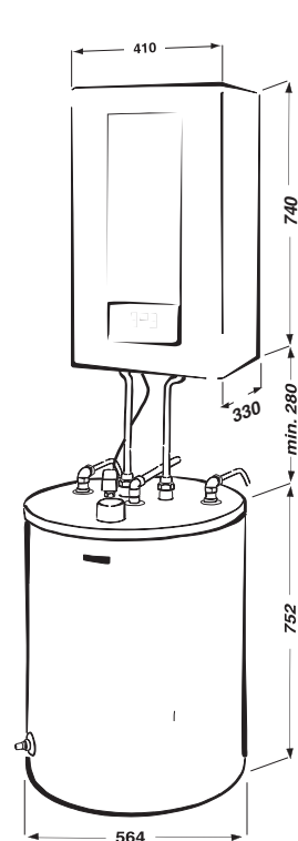
Rozmerový náčrtok zostavy Panther 24 KTO / KOO + B 120 S
