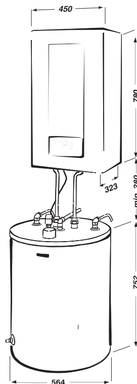
Rozmerový náčrtok zostavy Lev 28 KKO + B 120 S
