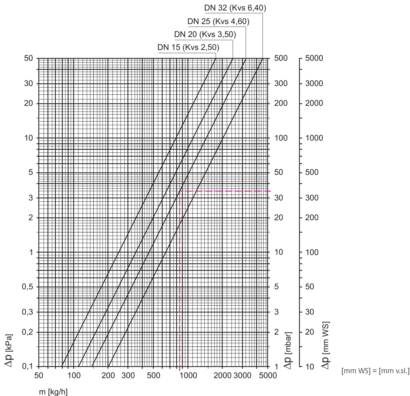
Diagram – Kvs hodnoty třícestných směšovacích ventilů
