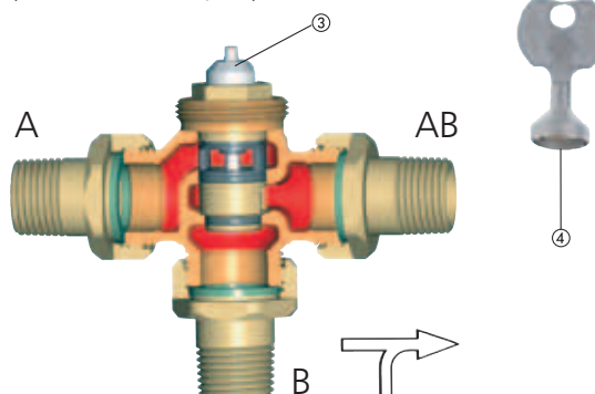
Třícestný směšovací ventil s nastavením (bílá ochranná krytka)
