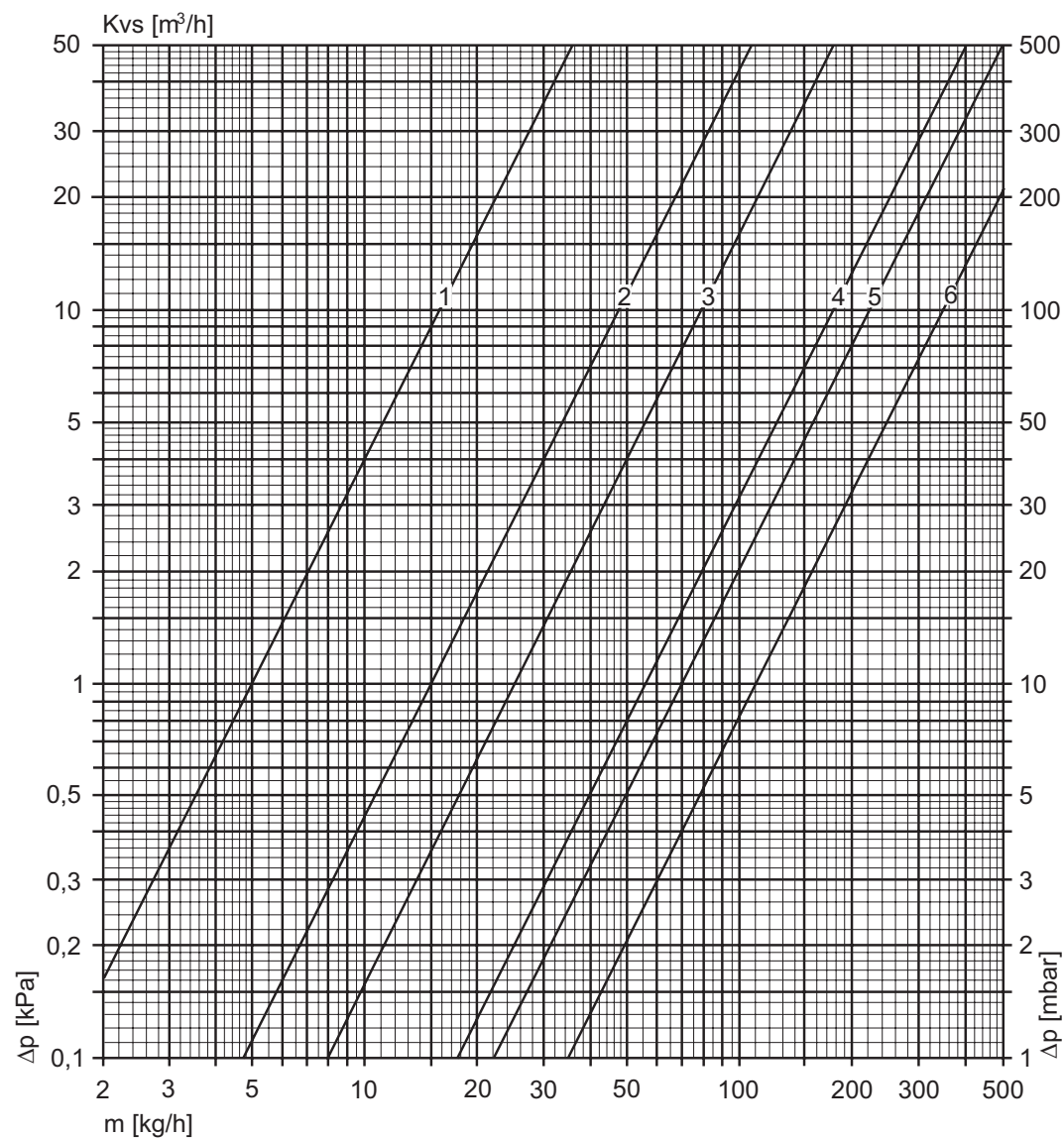
Diagram – Kvs hodnoty třícestných směšovacích ventilů s nastavením
