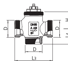
Kónicky těsnící
